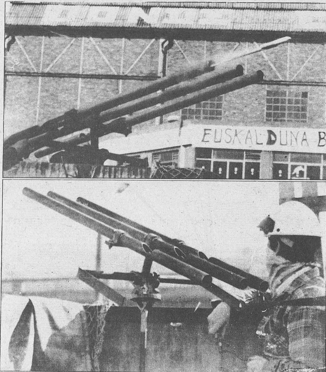
Artificio articulado de tres cañones fabricado por los trabajadores de Euskalduna con el que disparan cohetes, como demuestra la imagen superior.
