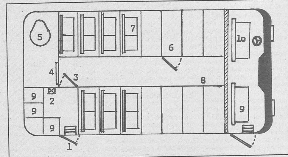
1: Puerta de entrada de los presos.—2: Mando neumático para apertura de las celdillas.—3: Puerta móvil.—4: Puerta de W. C.—5: W. C.—6: Celdillas.—7: Asientos de madera.—8: Rejilla de separación entre celdillas.—9: Asientos acolchados para la Guardia Civil.—9: Conductor.
